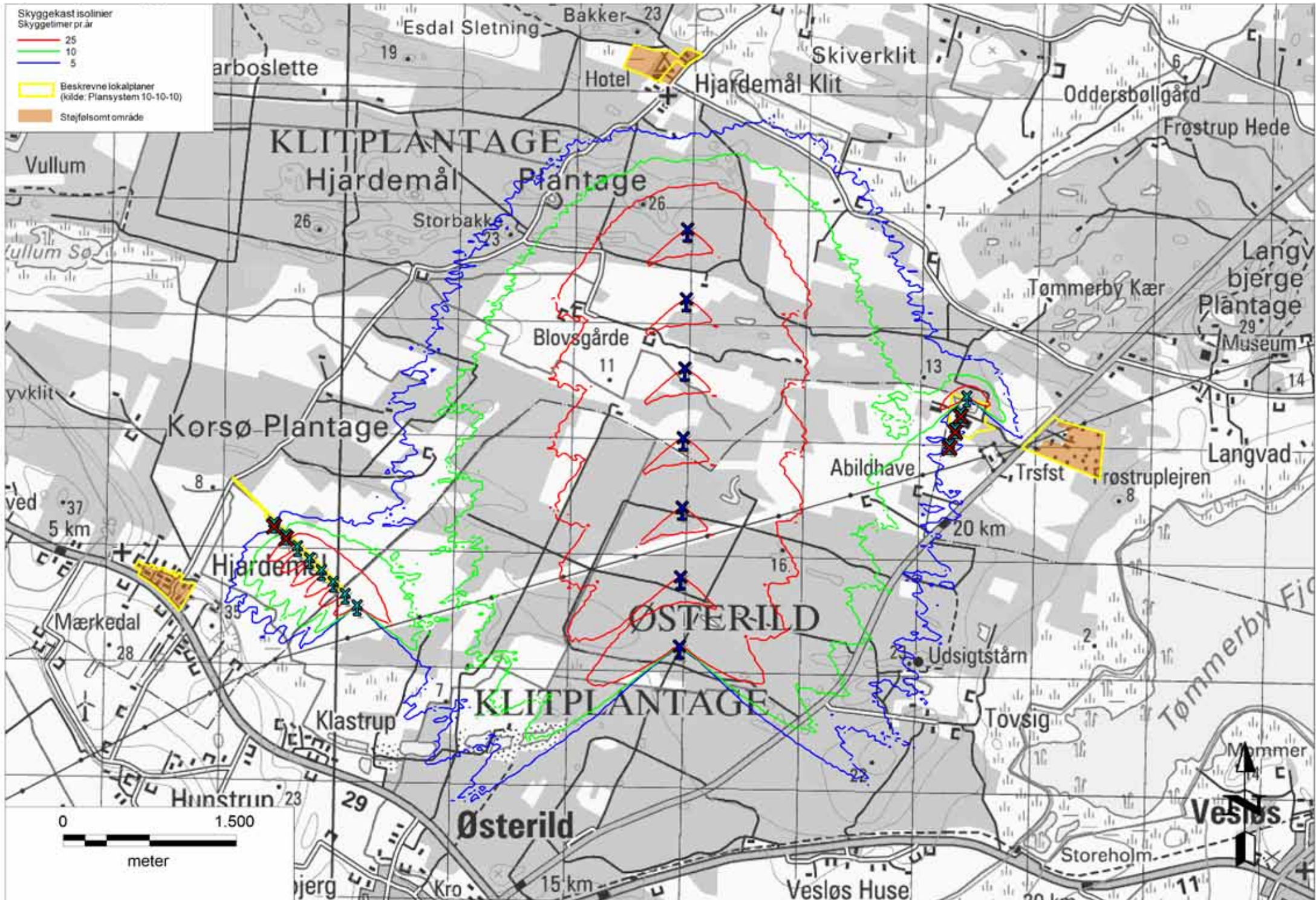
Figur 2A Isolinjer for reel skyggetid i timer pr. år.
