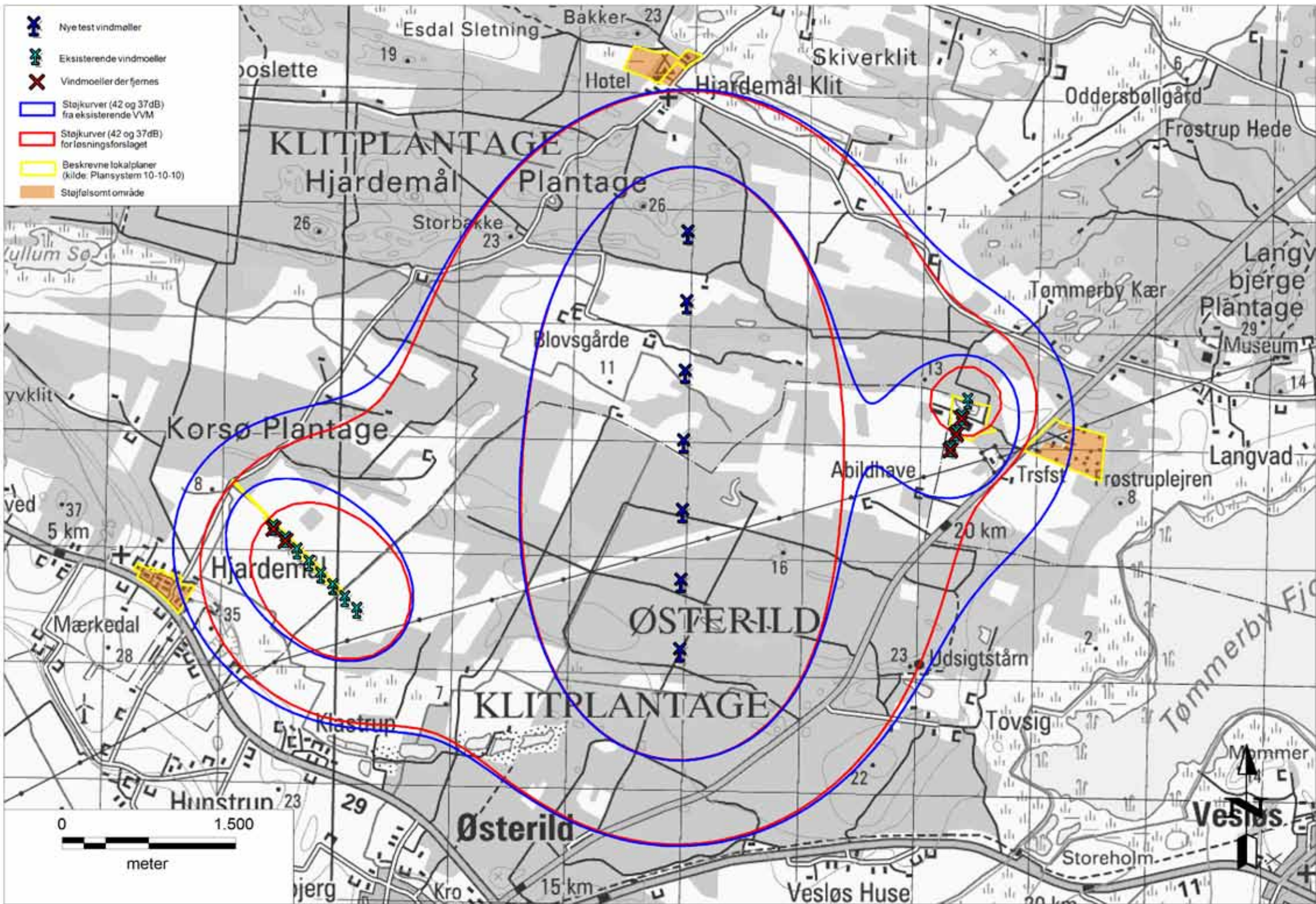
Figur 1A Støjkonsekvensområdet. Den beregnede støjkontur for 37 og 42dB ved 6 m/s for den samlede støj fra testcentret og de eksisterende vindmøller, der ikke nedtages.
