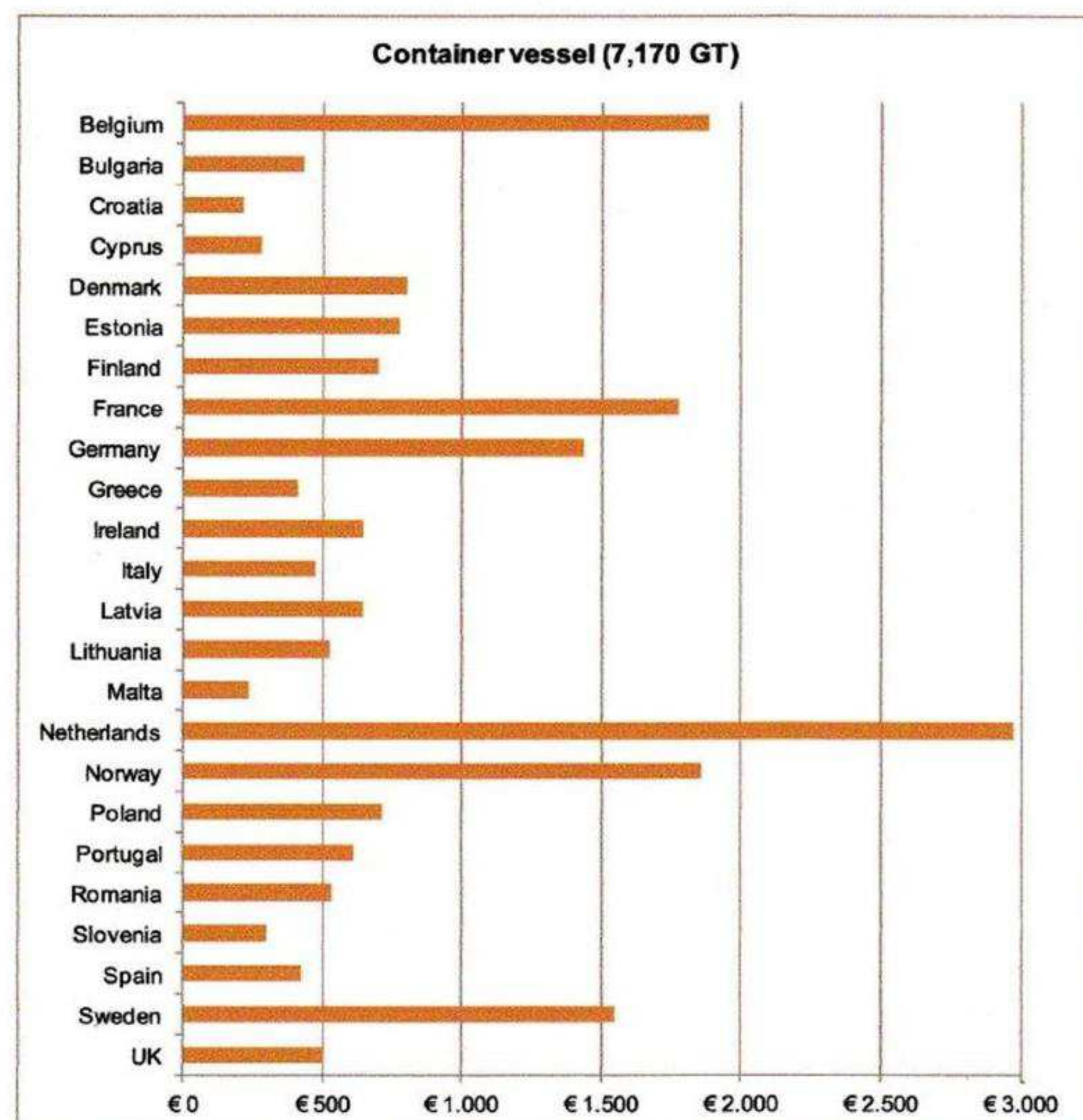
Figur 2 Gennemsnitlig pris for lodsning: Containerskib 5
